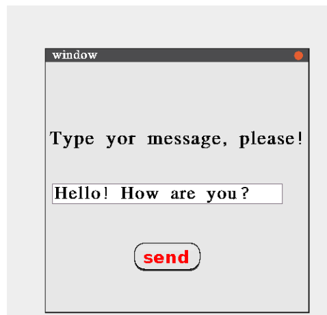
Рис. 12: Окно
