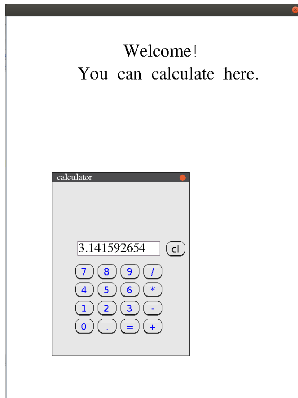
Рис. 19: Калькулятор
