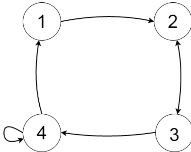
Рис. 18: Конечный автомат
