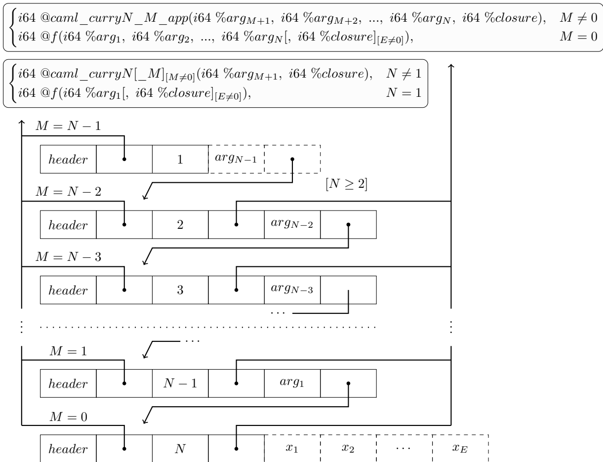
Рис. 1: Представление замыканий и частично применённых функций в OCaml
