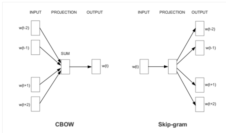
Рис. 2: Принцип работы алгоритма Word2Vec
